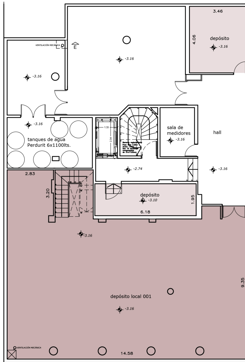
Subsuelo
