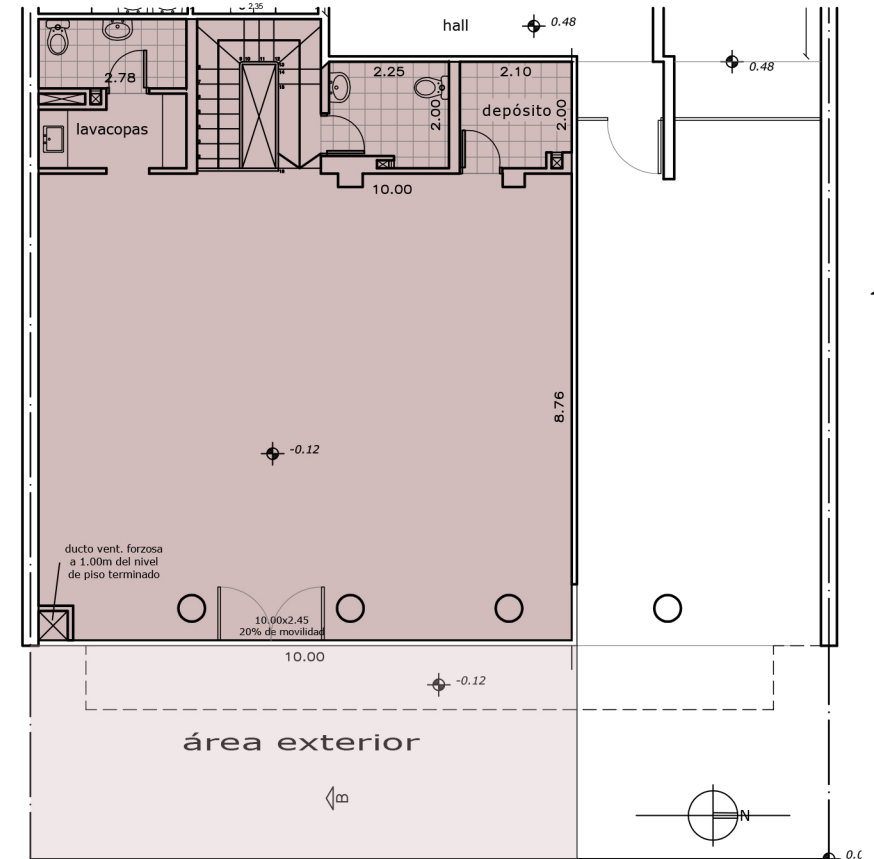
Planta Baja
